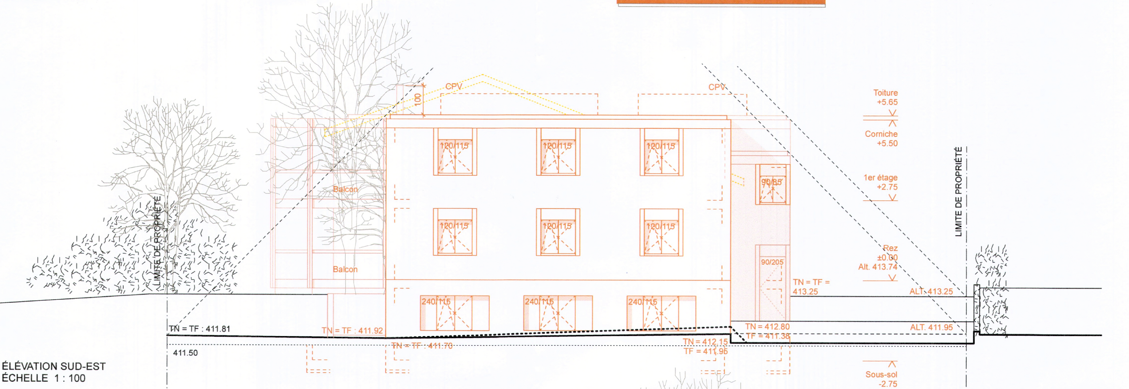
COUPE B-B ÉCHELLE 1 : 100
