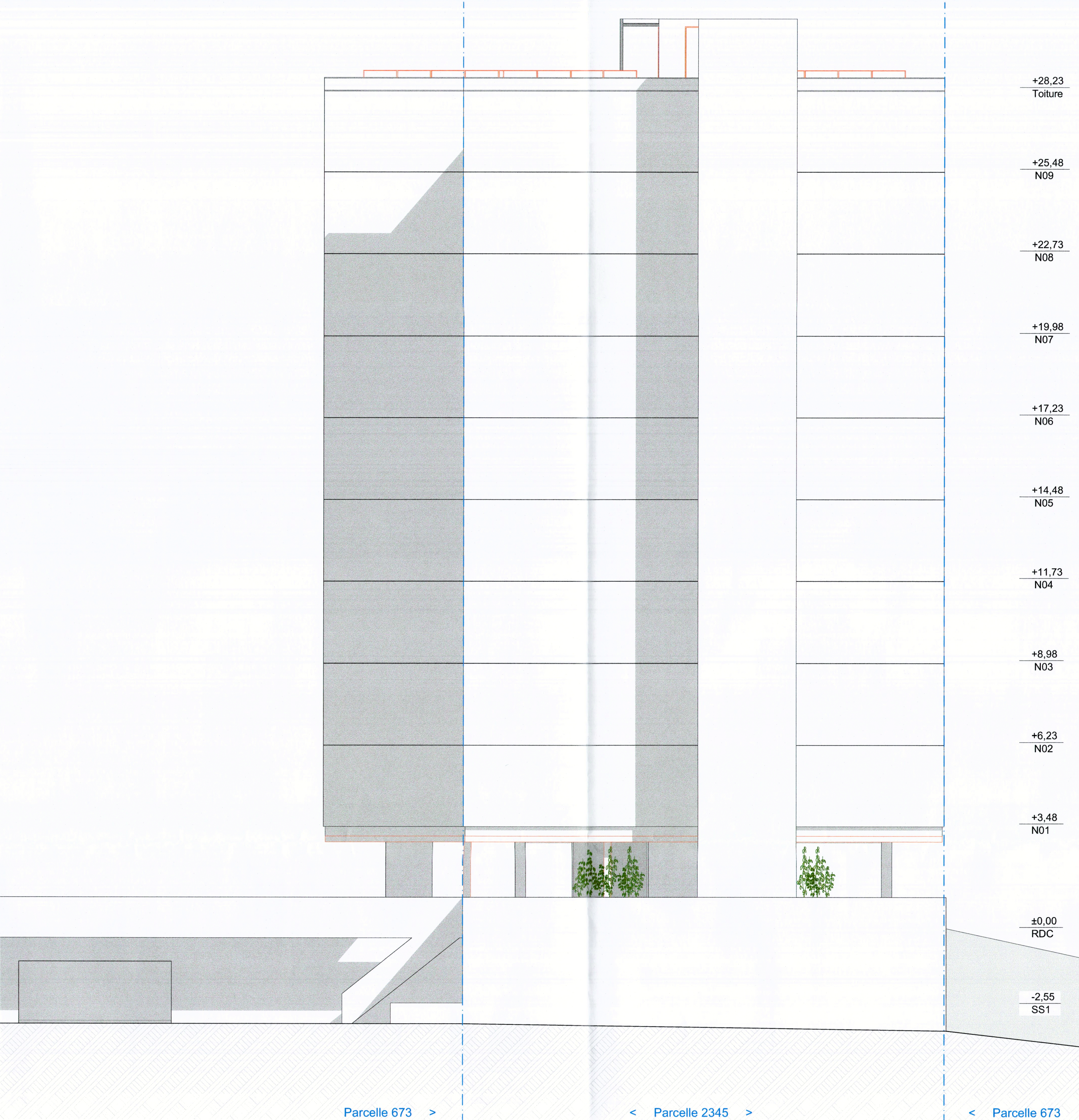
FAÇADE NORD
